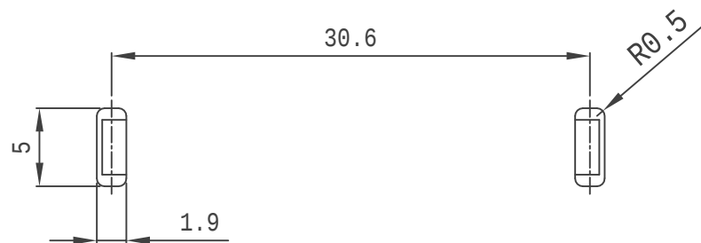
安装尺寸
