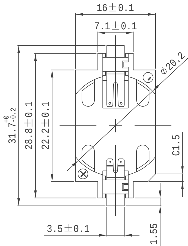
安装尺寸
